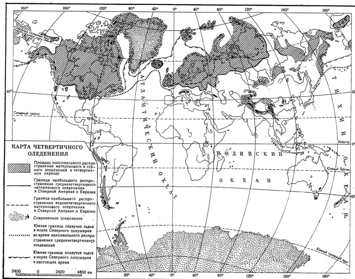
Рис. 2 – Плейстоценовые оледенения
