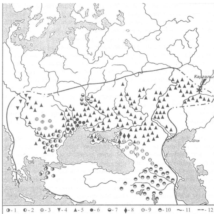
Северная часть Циркумпонтийской металлургической провинции в раннем бронзовом веке (по Е. Н. Черных с дополнениями Н. В. Рындиной). Схема расположения археологических памятников и очагов металлопроизводства: 1 - культура Трои I (очаг металлургии); 2 - культура Эзеро (очаг металлообработки); 3 - трансильванский очаг; 4 - культура Брно-Лишн-Евизовице; 5 - ямная общность (очаг металлургии и очаг металлообработки); 6 - усатовская культура (очаг металлообработки); 7 - софиевская культура (очаг металлообработки) ; 8 - новотитаровская культура; 9 - майкопская культура (очаг металлургии); 10 - куро-аракская культура (очаг металлургии); 11 - границы ЦМП; 12 - предполагаемые границы. (Рис. 33)[3].
